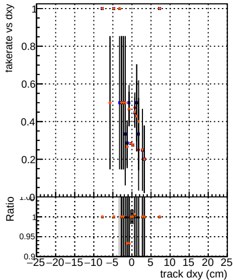
Fake rate vs d DQM IT original noPU DQM IT DQM IT MaxEffOnly FWD PU DQM IT DQM IT MaxEffOnly FWD PU
