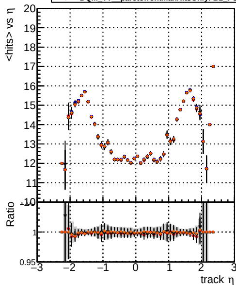
mean hit DQM TT original noPU DQM TT paretofrontMaxEffOnlyFB2_PU DQM TT paretofrontMinFOnlyFB2_PU DQM TT paretofrontMaxHitsOnlyFB2_PU
