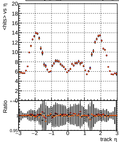
DQM TT original noPU DQM TT paretofrontMaxEffOnlyFB2_PU DQM TT paretofrontMinFROnlyFB2_PU DQM TT paretofrontMaxHitsOnlyFB2_PU
