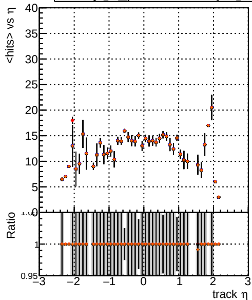
mean hit DQM TT original noPU DQM TT paretofrontMaxEffOnlyFB2_PU DQM TT paretofrontMinFB2_PU DQM TT paretofrontMaxHitsOnlyFB2_PU
