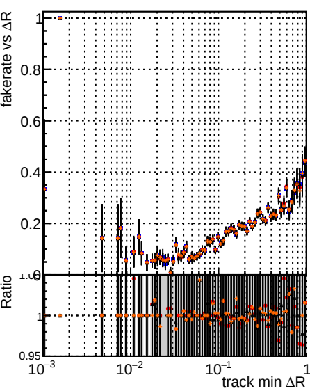
Fake rate vs \Delta R(\text{track, jet}) DQM TT original noPU DQM TT paretofrontMaxEffOnlyFB2_PU DQM TT paretofrontMinHitOnlyFB2_PU DQM TT paretofrontMaxHitOnlyFB2_PU
