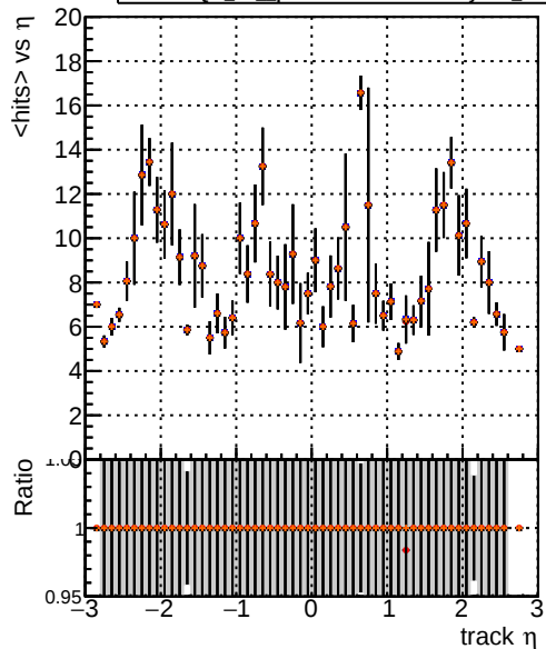
mean hits DQM TT original noPU DQM TT paretofrontMaxEffOnlyFB2_PU DQM TT paretofrontMinFB2_PU DQM TT paretofrontMaxHitsOnlyFB2_PU
