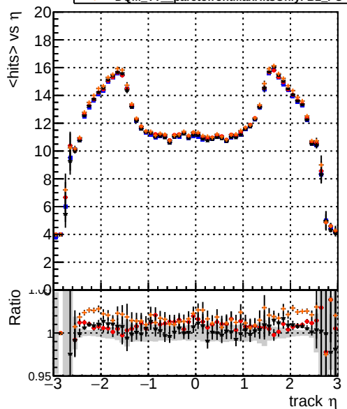
mean hits DQM TT original noPU DQM TT paretofrontMaxEffOnlyFB2_PU DQM TT paretofrontMinFROOnlyFB2_PU DQM TT paretofrontMaxHitsOnlyFB2_PU
