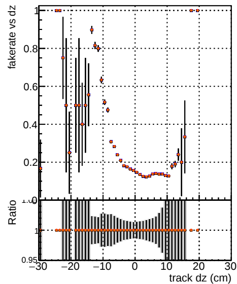
Fake rate vs dz Legend: original noPU original noPU + MaxEff original noPU + MaxEff + B2 PU original noPU + MaxEff + B2 PU + B2 PU original noPU + MaxEff + B2 PU + B2 PU + B2 PU original noPU + MaxEff + B2 PU + B2 PU + B2 PU + B2 PU original noPU + MaxEff + B2 PU + B2 PU + B2 PU + B2 PU + B2 PU original noPU + MaxEff + B2 PU + B2 PU + B2 PU + B2 PU + B2 PU + B2 PU original noPU + MaxEff + B2 PU + B2 PU + B2 PU + B2 PU + B2 PU + B2 PU + B2 PU original noPU + MaxEff + B2 PU + B2 PU + B2 PU + B2 PU + B2 PU + B2 PU + B2 PU + B2 PU
