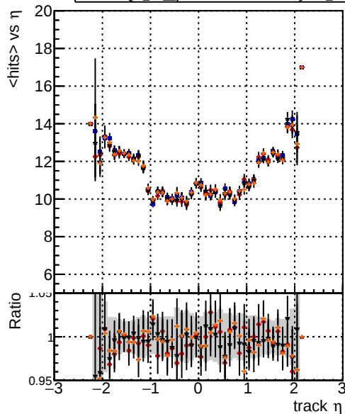
Legend: DQM TT original noPU DQM TT paretofrontMaxEffOnlyFB2_PU DQM TT paretofrontMinFROnlyFB2_PU DQM TT paretofrontMaxHitsOnlyFB2_PU
