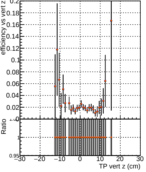
Efficiency vs vert z Legend: DQM TT original_noPU DQM TT paretofrontMaxEffOnlyFB2_PU DQM TT paretofrontMinFROnlyFB2_PU DQM TT paretofrontMaxHitsOnlyFB2_PU
