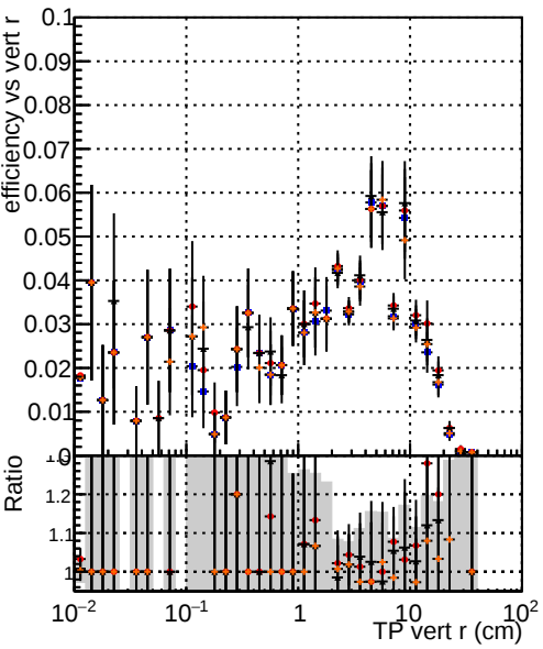
Efficiency vs TP vert r (cm) —•— DQM TT original noPU —•— DQM TT paretofrontMaxEff_PU —•— DQM TT paretofrontMaxHits_PU —•— DQM TT paretofrontMinFR_PU
