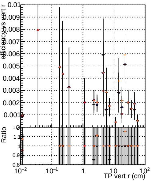
Efficiency vs TP vert r (cm) Legend: DQM TT original noPU DQM TT paretofrontMaxEff_PU DQM TT paretofrontMaxHits_PU DQM TT paretofrontMinFR_PU
