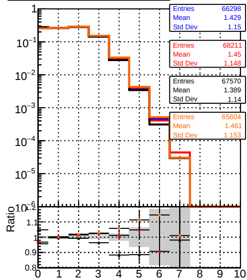
mean hits vs \eta DQM TT original noPU DQM TT paretofrontMaxEff_PU DQM TT paretofrontMaxHits_PU DQM TT paretofrontMinFR_PU
