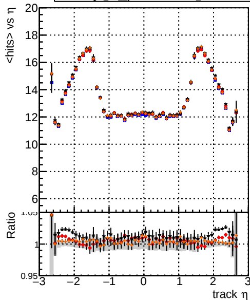
mean hits vs \eta DQM TT original noPU DQM TT paretofrontMaxEff_PU DQM TT paretofrontMaxHits_PU DQM TT paretofrontMinFR_PU
