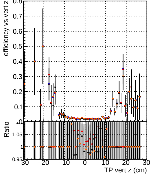
Efficiency vs. TP vert z (cm) —●— DQM TT original noPU —●— DQM TT paretofrontMaxEff_PU —●— DQM TT paretofrontMaxHits_PU —●— DQM TT paretofrontMinFR_PU
