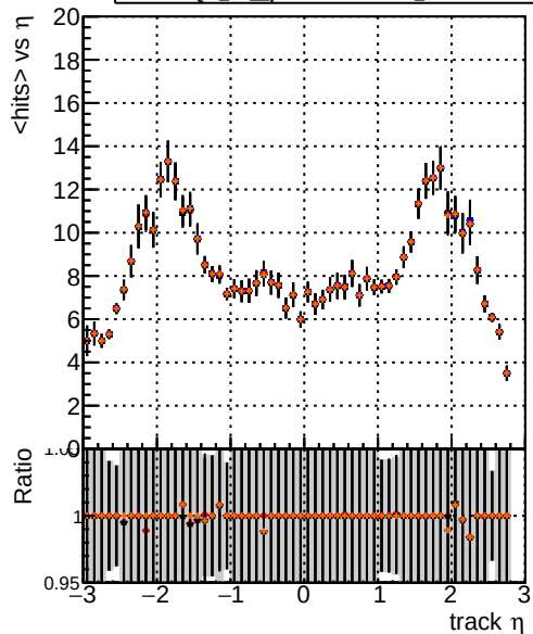
mean hit DQM TT original noPU DQM TT paretofrontMaxEff_PU DQM TT paretofrontMaxHits_PU DQM TT paretofrontMinFR_PU
