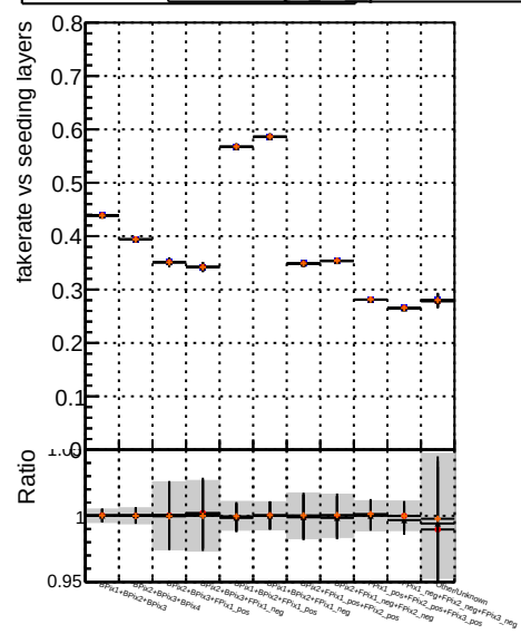
Fake rate vs. DGM TT original noPU pareto frontMax Eff PU frontMin Effs PU MinFR PU
