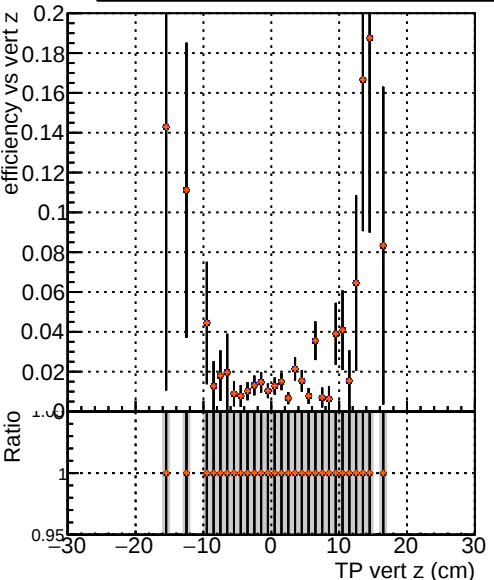
Efficiency vs vertpos —●— DQM TT original noPU —●— DQM TT paretofrontMaxEff_PU —●— DQM TT paretofrontMaxHits_PU —●— DQM TT paretofrontMinFR_PU
