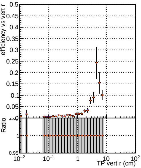
Efficiency vs vertpos —●— DQM TT original noPU —●— DQM TT paretofrontMaxEff_PU —●— DQM TT paretofrontMaxHits_PU —●— DQM TT paretofrontMinFR_PU
