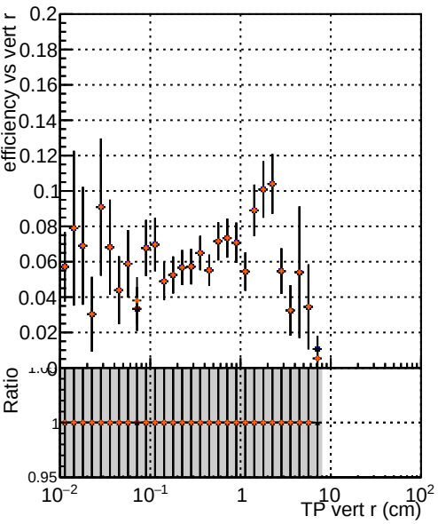
Efficiency vs vertpos Legend: — DQM TT original noPU — DQM TT paretofrontMaxEff_PU — DQM TT paretofrontMaxHits_PU — DQM TT paretofrontMinFR_PU
