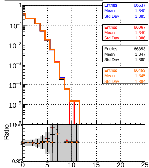
mean hits DQM TT original noPU DQM TT paretofrontMaxEff_PU DQM TT paretofrontMaxHits_PU DQM TT paretofrontMinFR_PU
