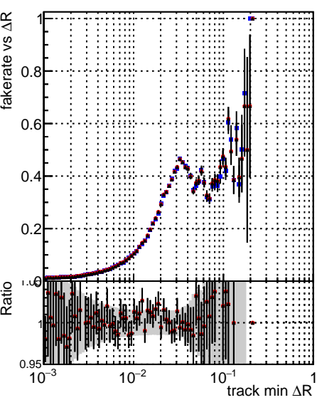
—•— DQM TT original —•— DQM TT initOnlyFWD0_PU —•— DQM TT initOnlyFWD0_PU
