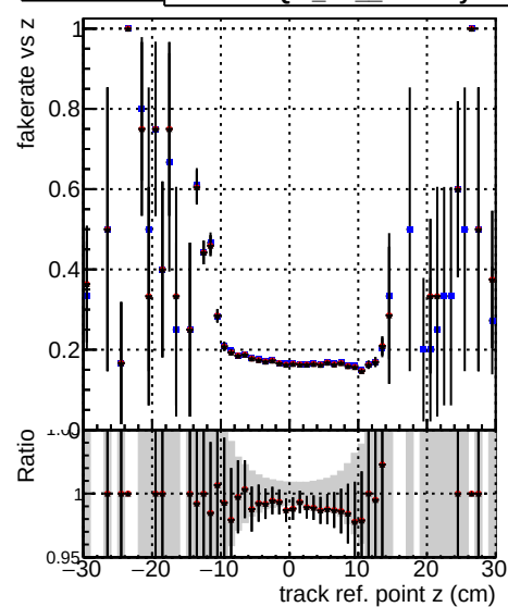
—●— DOM TT original —●— DOM TT initOnlyFWD0 —●— DOM TT initOnlyFWD0 PU
