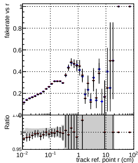
—●— DOM TT original —●— DOM TT initOnlyFWD0 —●— DOM TT initOnlyFWD0 PU
