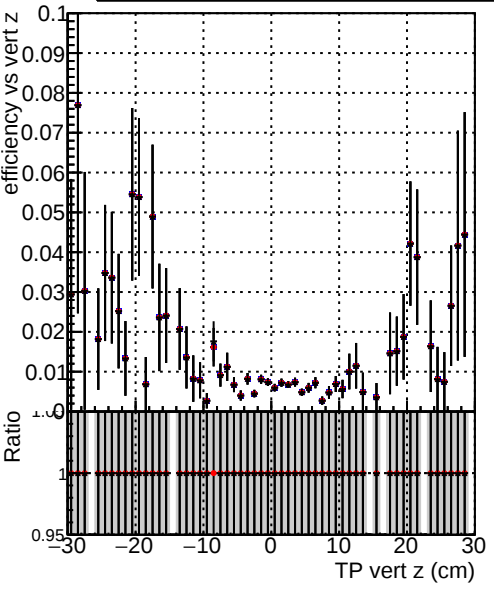
Efficiency vs TP vert z (cm) Legend: DQM_TT_original DQM_TT_detQ0_PU DQM_TT_detQ1_PU
