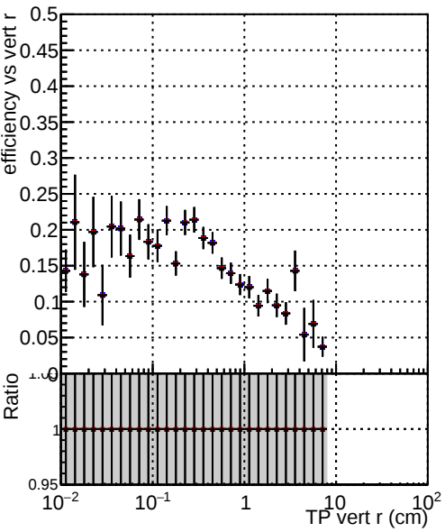
Efficiency vs TP vert r (cm) DQM_TT_original DQM_TT_detQ0_PU DQM_TT_detQ1_PU
