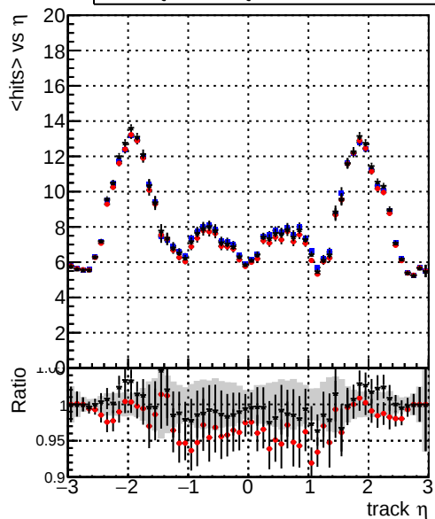
mean hit — DQM_TT_original — DQM_TT_detQ0_PU — DQM_TT_detQ1_PU
