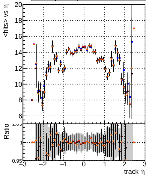
mean hit — DQM TT original — DQM TT 0pt09 PU — DQM TT 1pt09 PU — DQM TT 2pt09 PU
