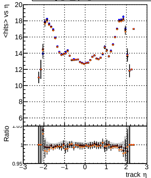
DQM TT original DQM TT 0pt09_PU DQM TT 1pt09_PU DQM TT 2pt09_PU mean hit
