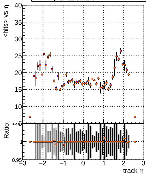
— DQM TT original — DQM TT 0pt09_PU — DQM TT 1pt09_PU — DQM TT 2pt09_PU mean hit
