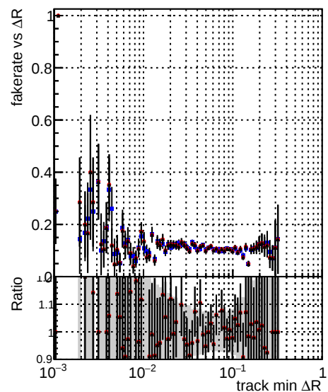
—•— DOM TT original —•— DOM TT Opt109 PU3 —•— DOM TT 1pt109 PU3
