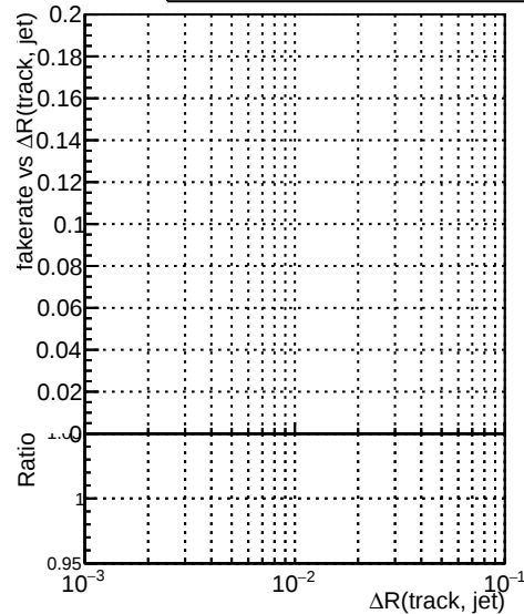
—•— DOM TT original —•— DOM TT Opt109 PU3 —•— DOM TT 1pt109 PU3
