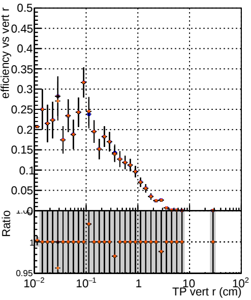
Efficiency vs vertpos —•— DQM TT original —•— DQM TT 0pt09_PU3 —•— DQM TT 1pt09_PU3 —•— DQM TT 2pt09_PU3
