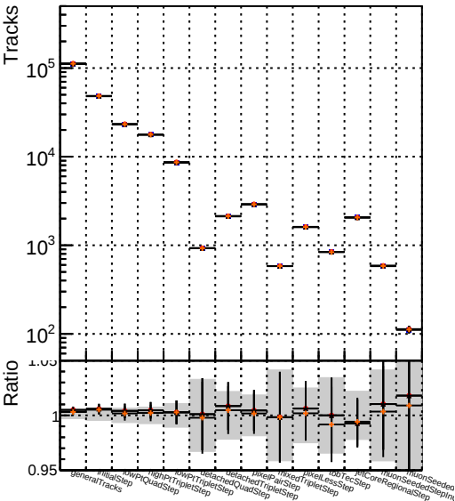
Number —■— DQM TT original —●— DQM TT 0pt09_PU3 —▲— DQM TT 1pt09_PU3 —★— DQM TT 2pt09_PU3
