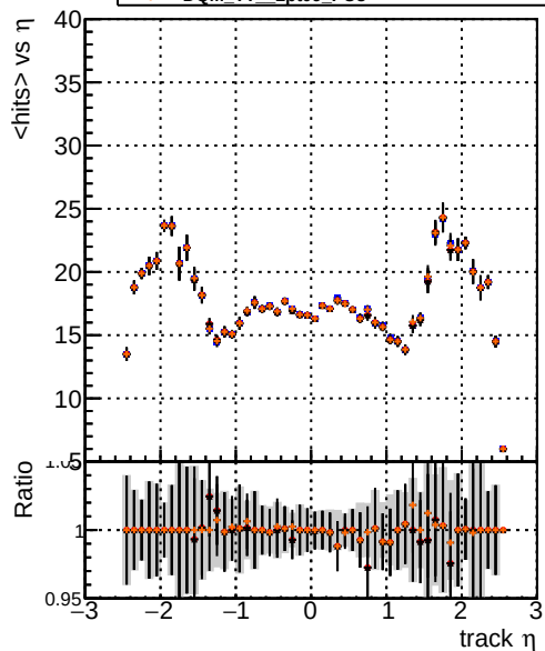
mean hit DQM TT original DQM TT 0pt09_PU3 DQM TT 1pt09_PU3 DQM TT 2pt09_PU3
