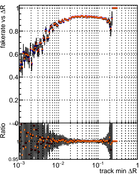
Fake rate vs —●— DQM TT original —●— DQM TT PU3 —●— DQM TT PU9
