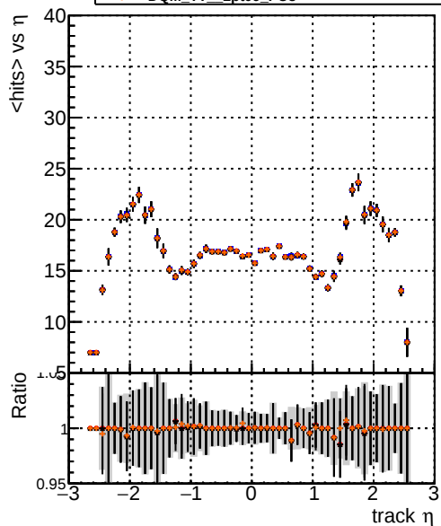
mean hits vs \eta DQM TT original DQM TT 0pt09_PU3 DQM TT 1pt09_PU3 DQM TT 2pt09_PU3
