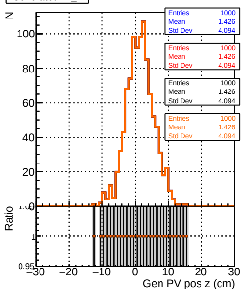
GeneratedPV_Z
