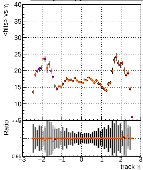
DQM TT original DQM TT 0ptg09 PU2 DQM TT 1ptg09 PU2 DQM TT 2ptg09 PU2 mean hits
