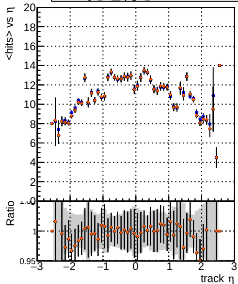
mean hit DQM TT original DQM TT 0ptg09_PU2 DQM TT 1ptg09_PU2 DQM TT 2ptg09_PU2
