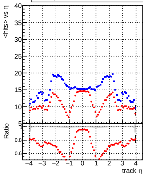
mean hits — DQM_CKF — DQM_mkFitnIt
