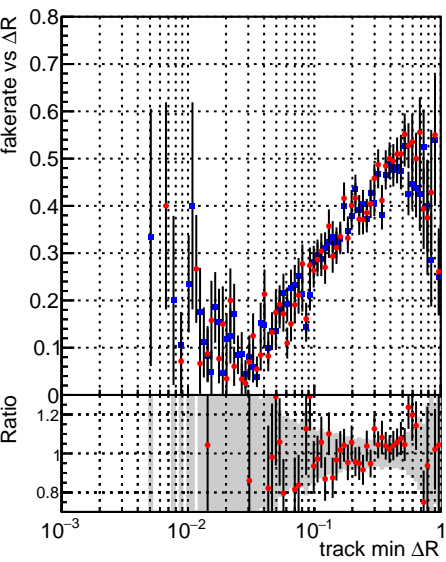
Fake rate vs \Delta R(\text{track, jet}) ■ DQM_CKF ■ DQM_mkFitInit
