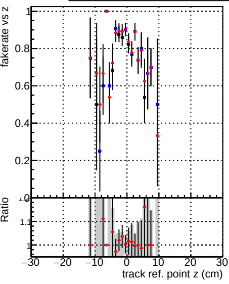
Fake rate vs v DQM_CKF DQM_mkFitlnit
