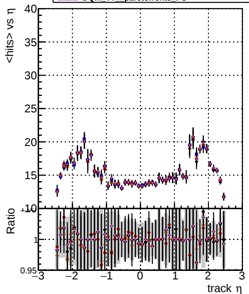
mean hit DOM TT original DOM TT paretofront4 PU DOM TT paretofront5 PU DOM TT paretofront6 PU DOM TT paretofront8 PU
