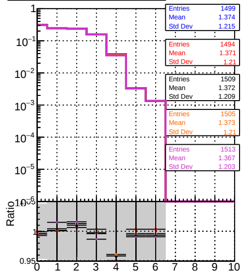
mean hit DOM TT original DOM TT paretofront4 PU DOM TT paretofront5 PU DOM TT paretofront6 PU DOM TT paretofront8 PU
