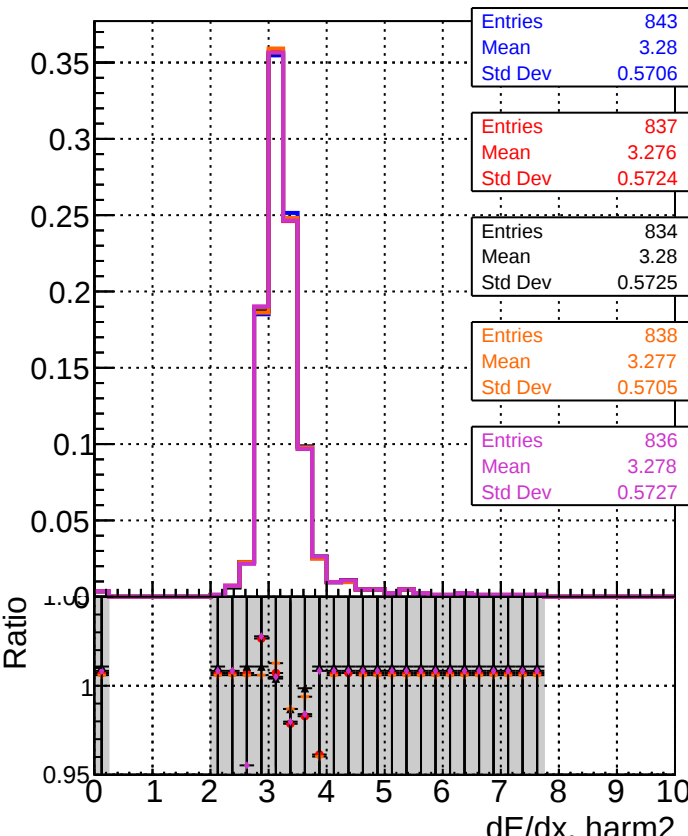
dE/dx estimator 1
