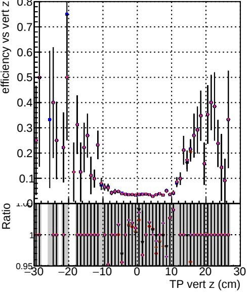
Efficiency vs. TP vert z (cm) DOM TP Method original PU original paretofront0 PU paretofront0 paretofront1 PU paretofront1 paretofront2 PU paretofront2 paretofront3 PU paretofront3
