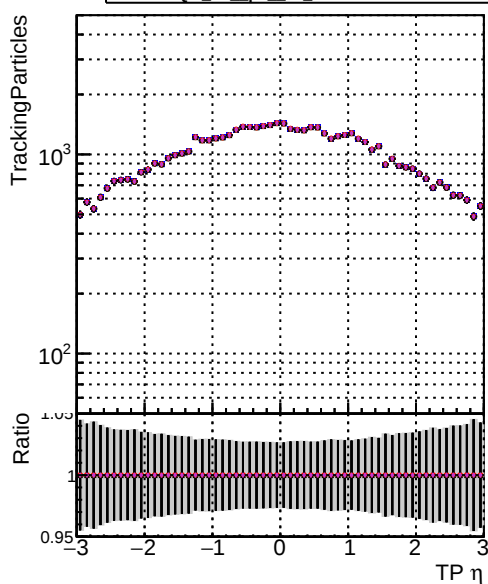
N of sim DOM TT pL 21 PU DOM TT pL 22 PU DOM TT pL 23 PU
