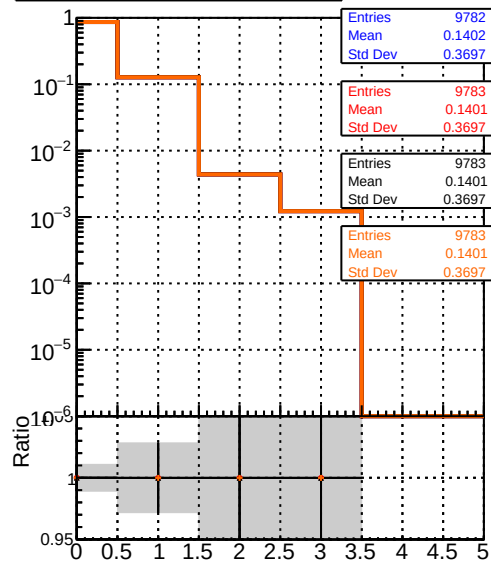
mean hits vs \eta Legend: - DQM TT original PU - DQM TT pL_eta3_1PU - DQM TT pL_eta3_2PU - DQM TT pL_eta3_2PU
