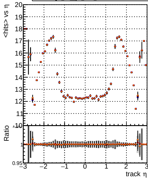
- - DQM TT original PU - - DQM TT pL_eta3_1PU - - DQM TT pL_eta3_2PU - - DQM TT pL_eta3_2PU
