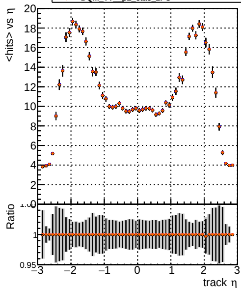
mean hit - - DQM TT original PU - - DQM TT pL_eta3_1PU - - DQM TT pL_eta3_2PU
