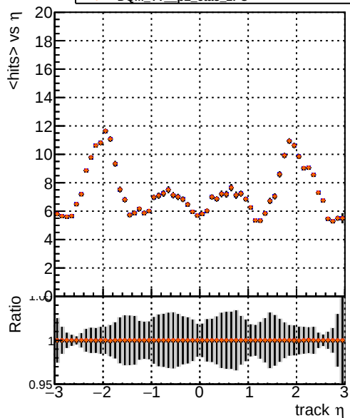
mean hits - - DQM TT original PU - - DQM TT pL_eta3_1PU - - DQM TT pL_eta3_2PU - - DQM TT pL_eta3_2PU
