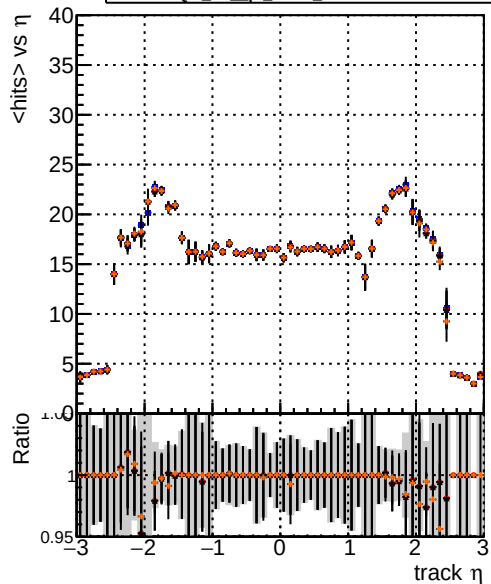
mean hits DQM TT original PU DQM TT pf eta25 1PU DQM TT pf eta25 2PU DQM TT pf eta25 3PU
