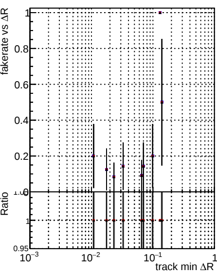
Fake rate vs \Delta R(\text{track, jet}) DQM TT originalREDO100 DQM TT originalREDO100f DQM TT originalREDO100f
