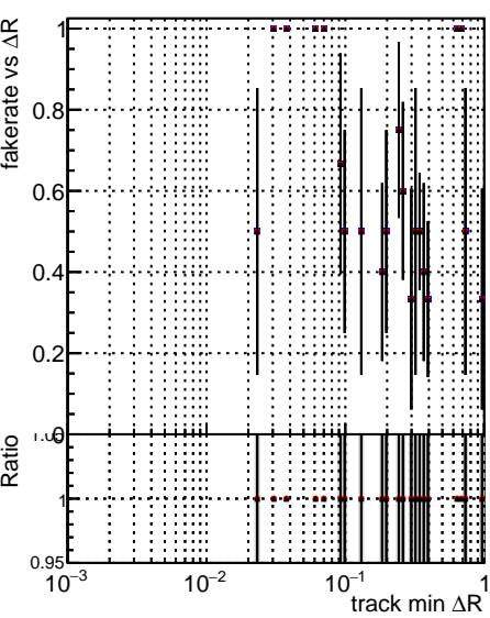
Fake rate vs —●— DQM TT originalREDO100 —●— DQM TT originalREDO100f —●— DQM TT originalREDO100f
